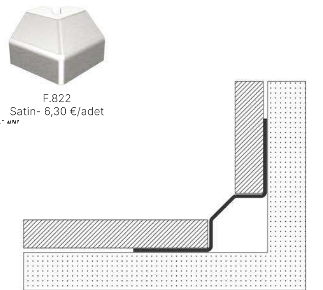
Dış Köşe
