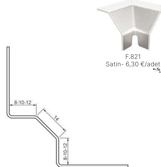
İç Köşe
