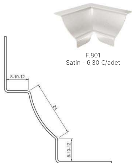
İç Köşe
